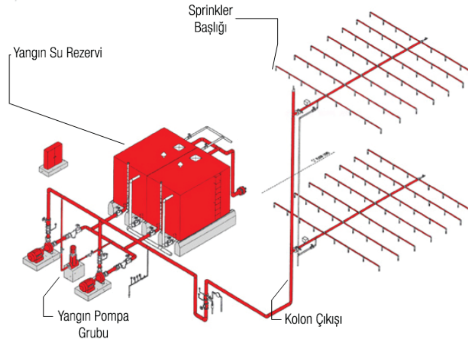
Sprinkler Tesisatı Uygulaması
