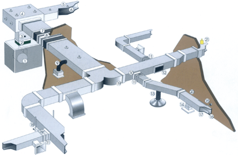
Havalandırma Kanalı Uygulaması
